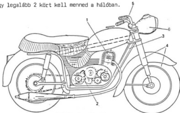
75. ábra. A motorkerékpár fő részei 1. motor, 2. sebesség-berendezés, 3. becsapós, 4. futómű, 5. kormány, 6. világítás
